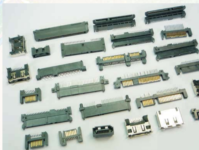
Serial ATA Connectors Series SATA 连接器系列
