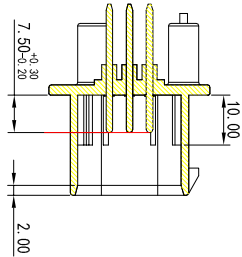
剖面A-A
