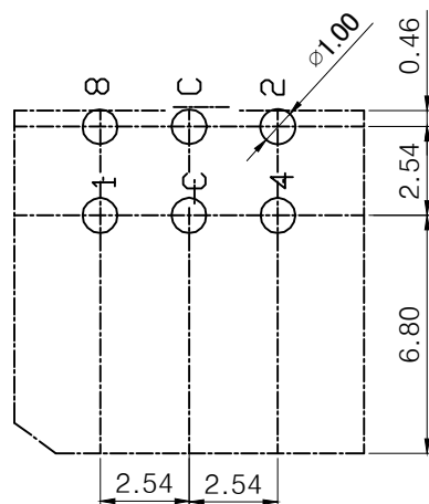
P.C.B Dimension
